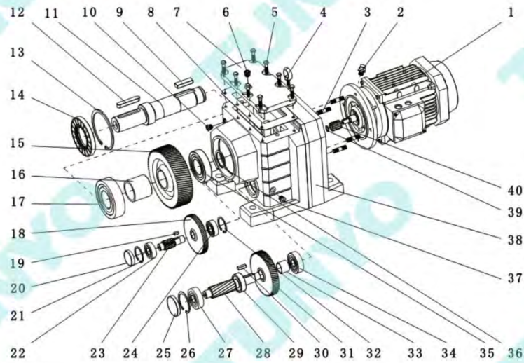
部件分解圖 Spare Parts List
