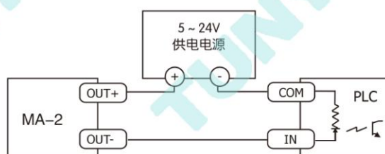
源电流输出的连接方式
