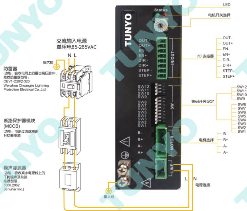
MA-2 接线图
