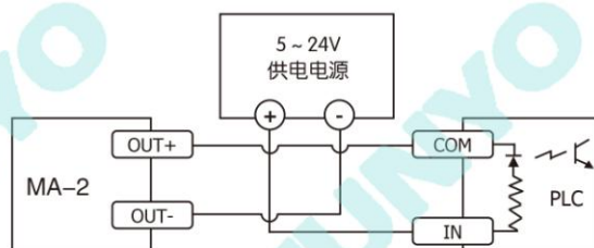
源电流输出连接PLC的方式
