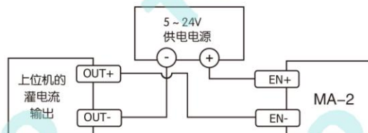
上位机的灌电流输出连接方式
