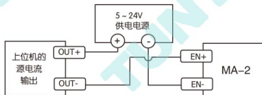
上位机的源电流输出连接方式
