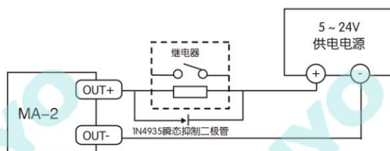
驱动一路继电器的连接方式
