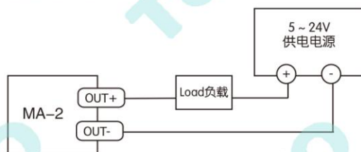
灌电流输出的连接方式
