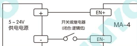
使用开关或继电器的连接方式
