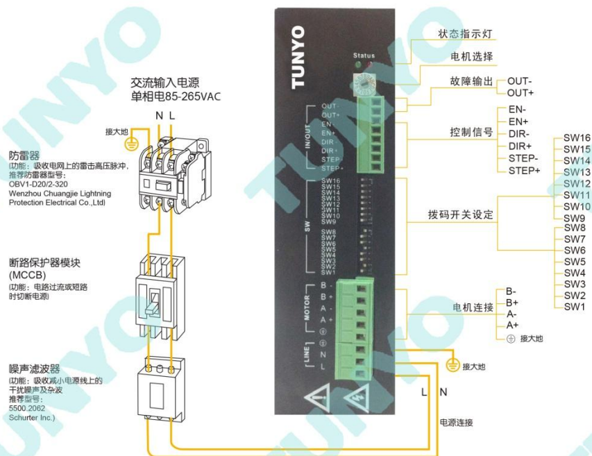
MA-4 接线图
