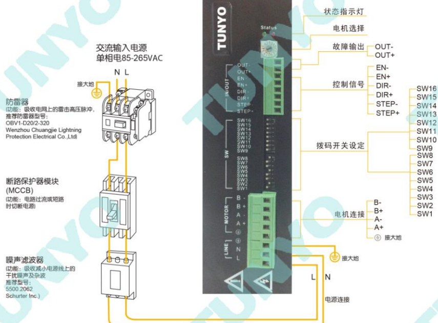
MA-8接线图
