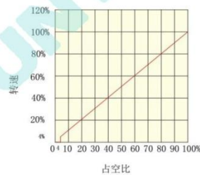
占空比与电机转速的关系（开环空载）
