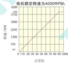
占空比与电机转速的关系（闭环空载）
